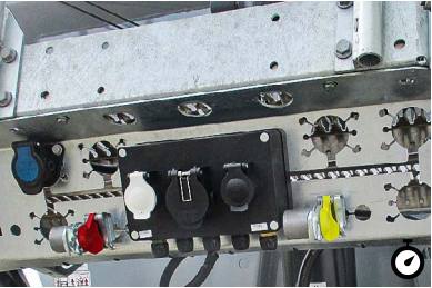
10 Fék- és világításcsatlakozók A fék- és világításcsatlakozók az elektromos és hidraulikus csatlakozókkal együtt kompakt és átlátható módon a jármű homlokfalán helyezkednek el.
