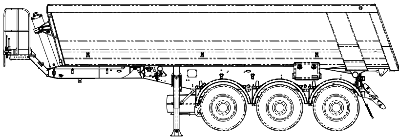
3-osý sklápěcí návěs se segmentovou korbou
