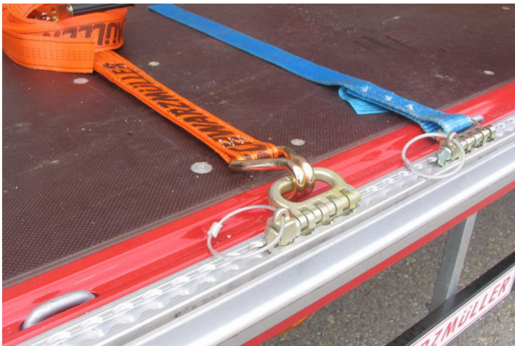
Rama zewnętrzna z wpuszczonymi uchwytami mocującymi 2,5 t
