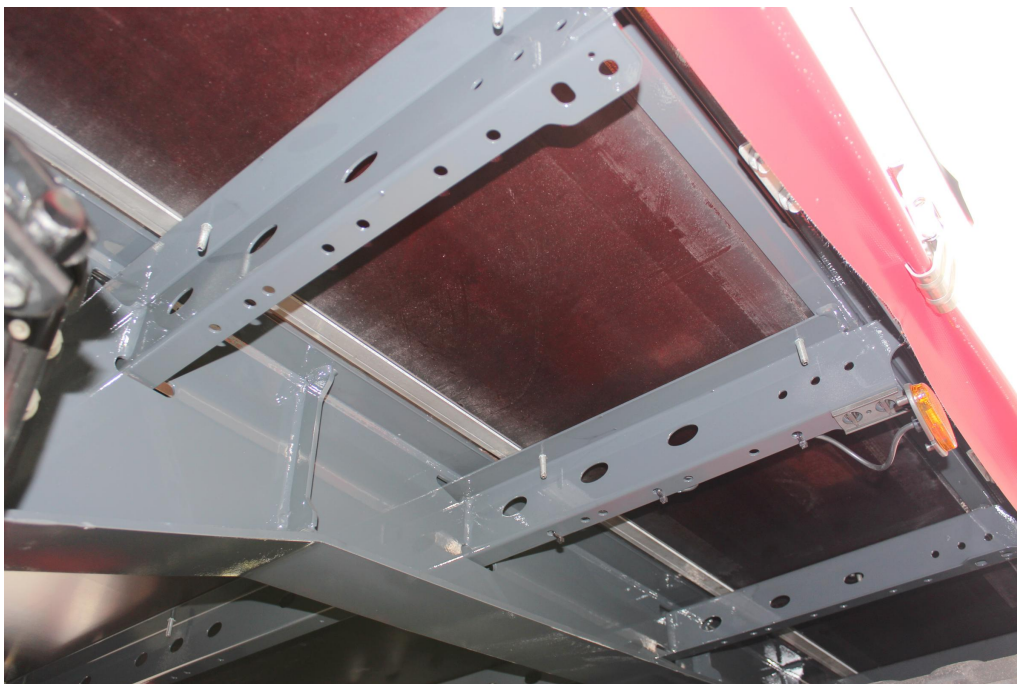
Odporna na skręcanie spawana konstrukcja ramy drabinowej
