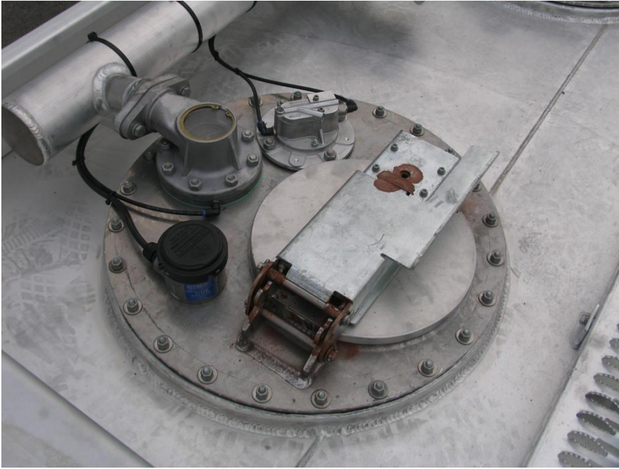
Przyjazne dla użytkownika rozmieszczenie armatury na włązie
