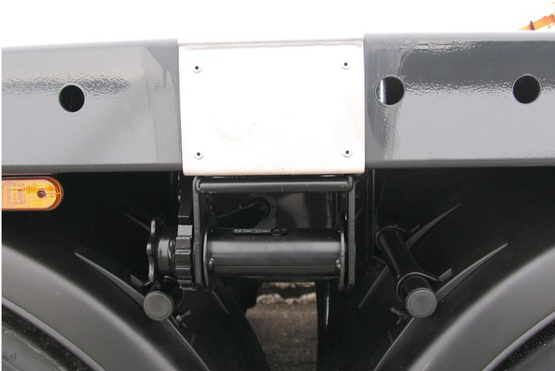
Łącznie 6 szt. wciągarek mocujących z liną drucianą, z blachami ciernymi ze stali szlachetnej na ramie zewnętrznej
