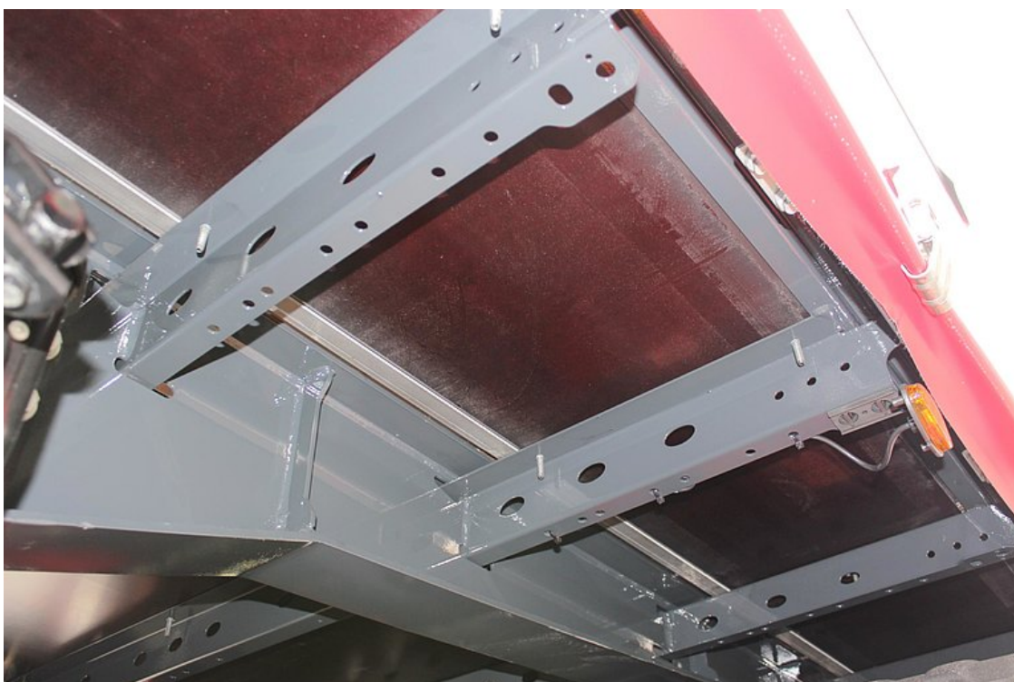
Podłoga ze sklejki wodoodpornej antypoślizgowej 27 mm, zlicowana z ramą zewnętrzną oraz 2 stalowe szyny profilowe nad podłużnicami (nacisk na oś wózka widłowego 7 t)
