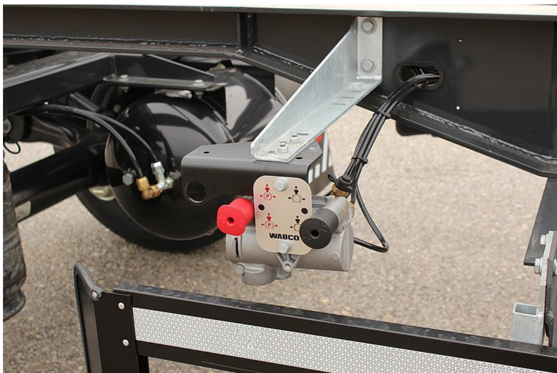
Zawór hamulcowy i zawór odłączający zamontowane z boku pojazdu, dla łatwej obsługi
