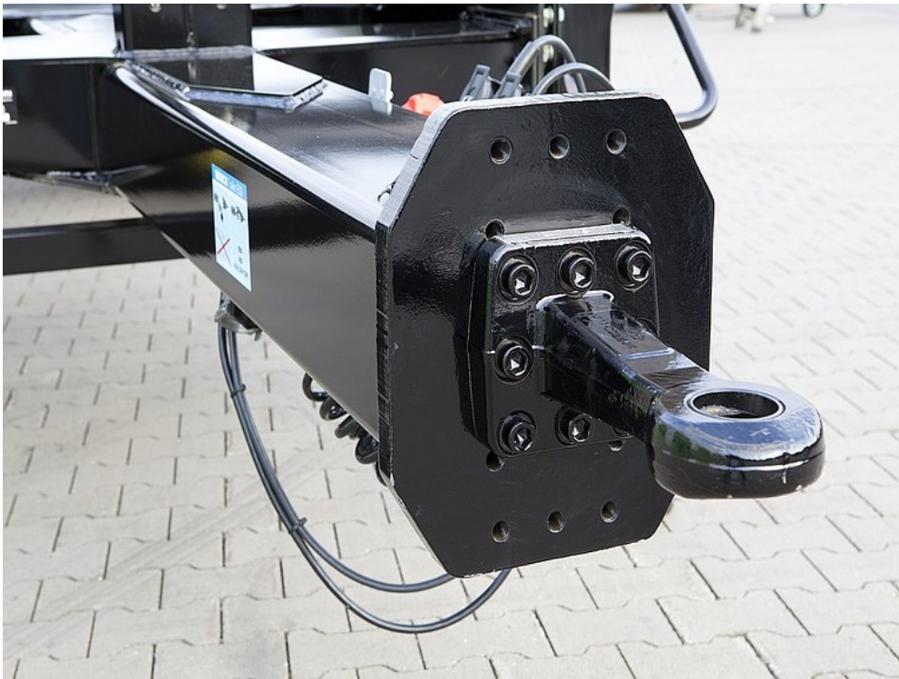
Spawany centralnoosiowy mechanizm pociągowy
