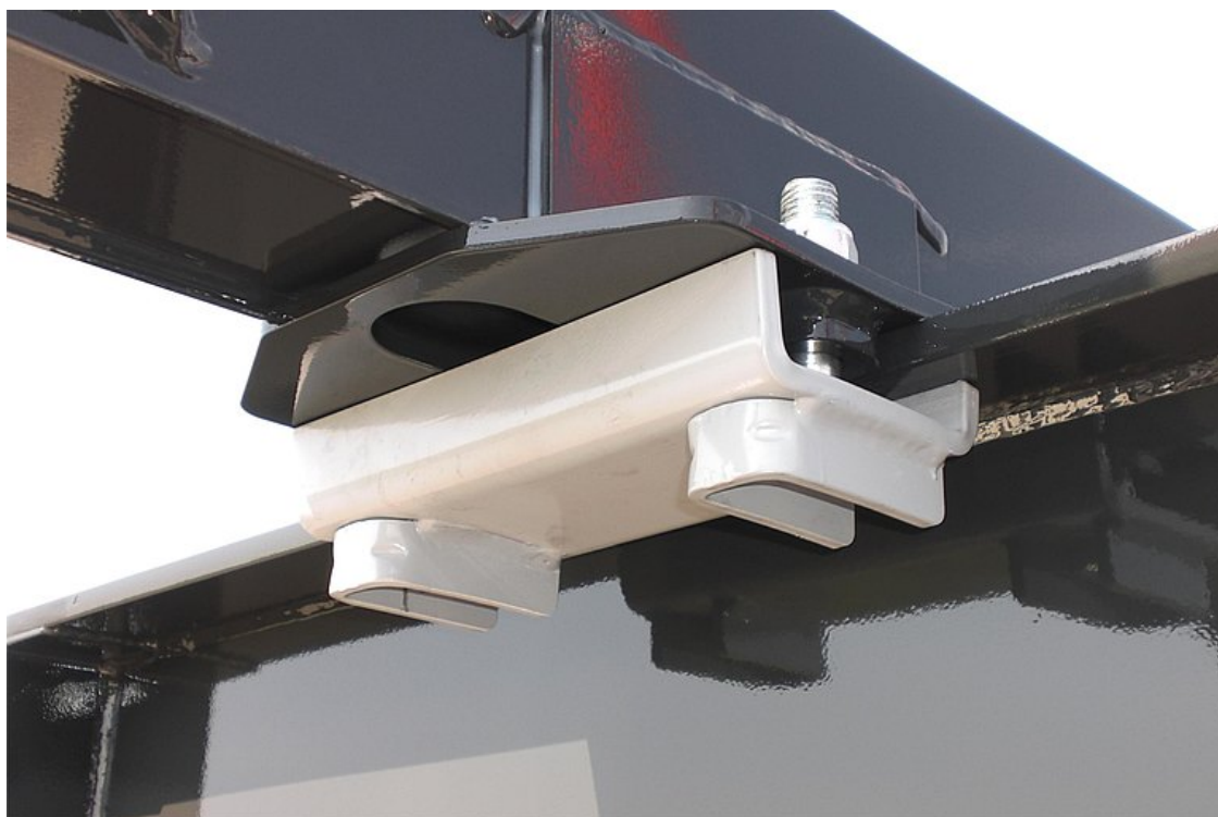
Słupki kłonic nasadzane za pomocą przyspawanych mocowań zaciskowych = mogą być przemieszczane
