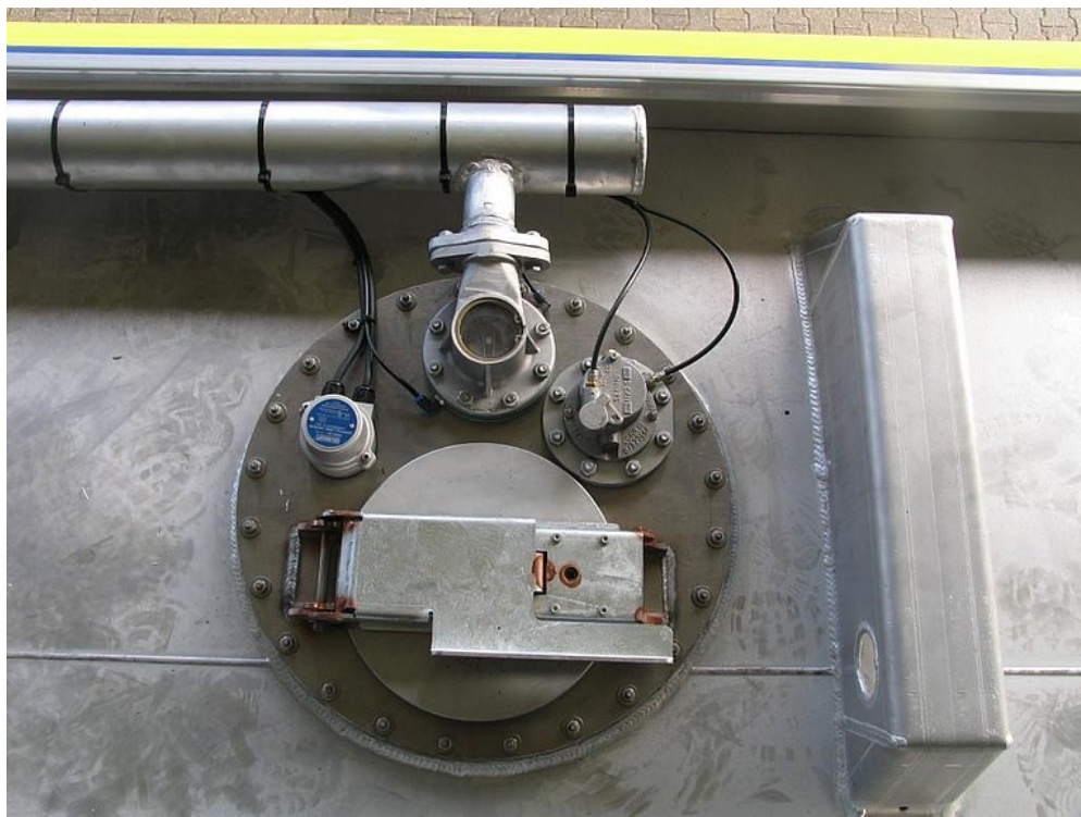
Przyjazne dla użytkownika rozmieszczenie armatury na włazie
