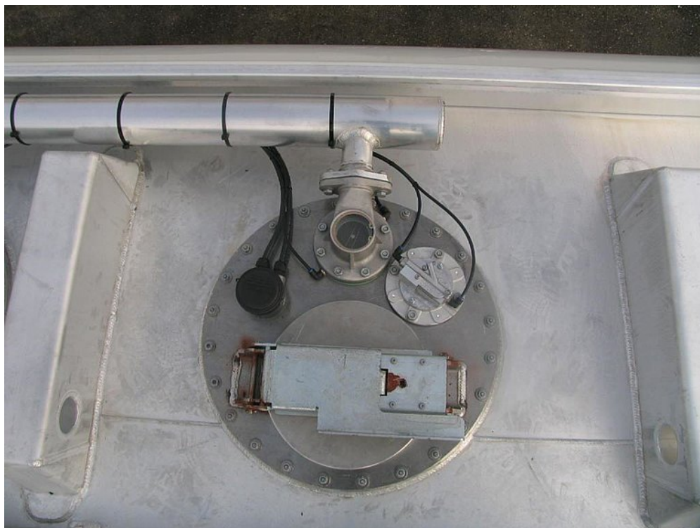
Przyjazne dla użytkownika rozmieszczenie armatury na wlocie
