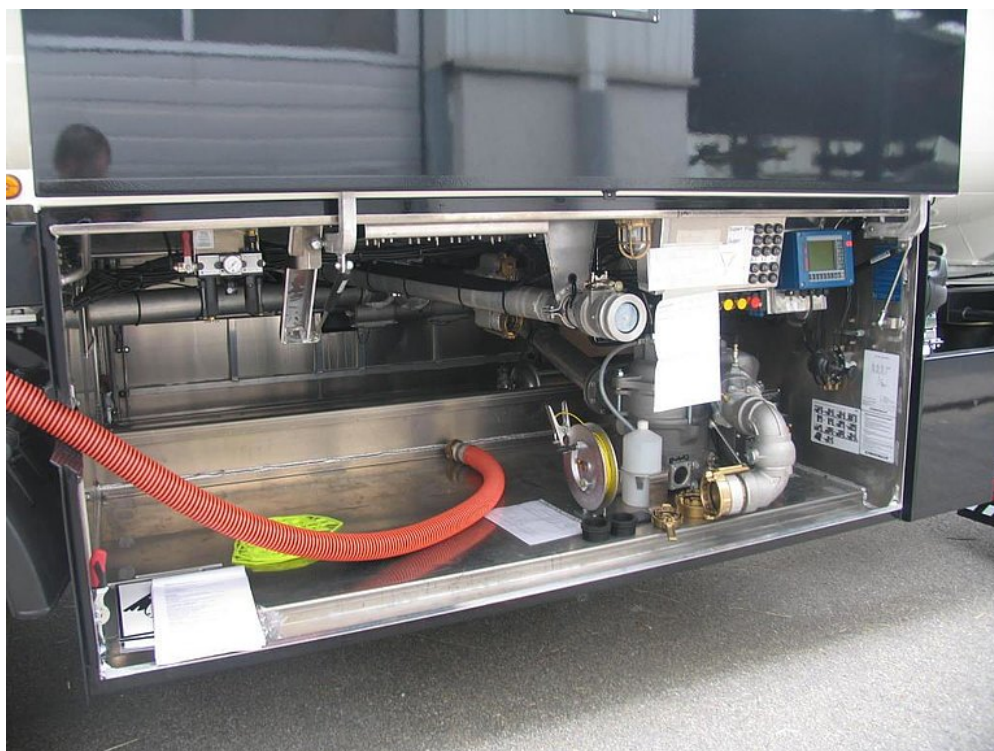
Przejrzyste i uporządkowane rozmieszczenie armatury zapewniające wydajną i bezawaryjną obsługę
