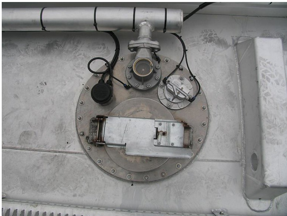
Przyjazne dla użytkownika rozmieszczenie armatury na włączniku
