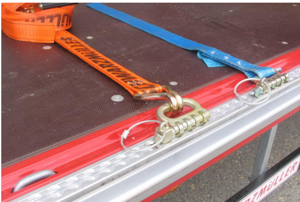
Lekötőgyűrűs keretszegély süllyesztett 2,5 t lekötőgyűrűv
