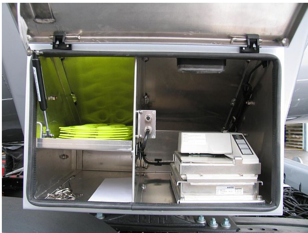
Elkülönített, nyomtató védelmére szolgáló láda, a fizikai behatások és időjárási viszonyok ellen
