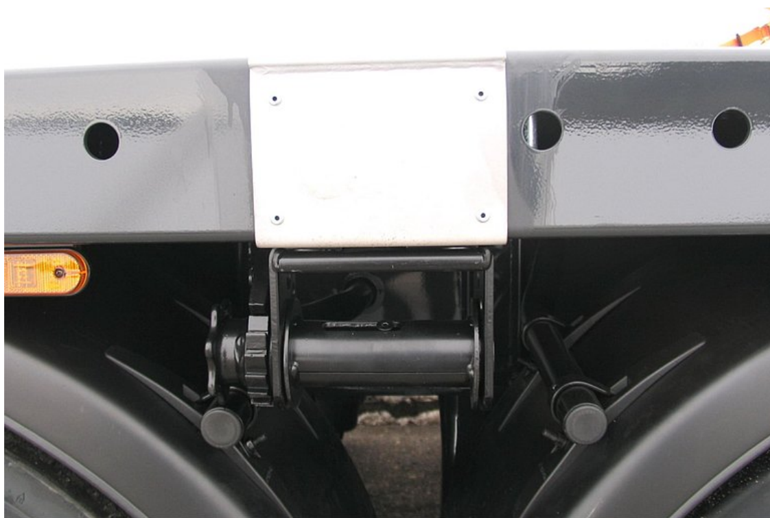
Összesen 6 db feszítő-csörlő kötéllal, rozsdamentes acél koptatóval a keretszegélyen
