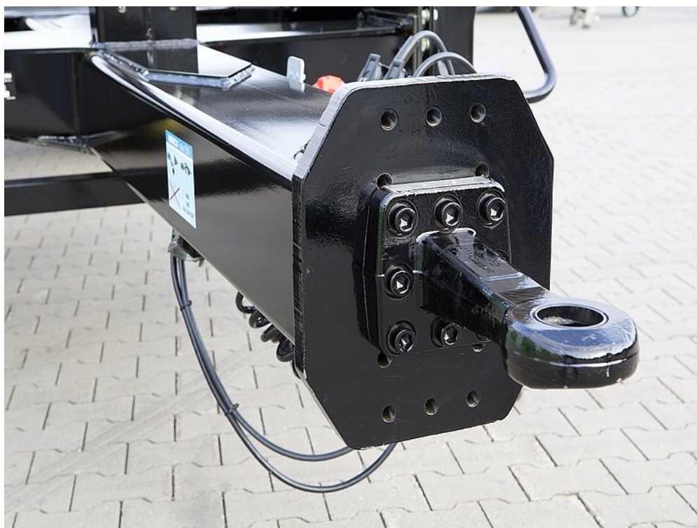
Hegesztett középső rudas vonóberendezés
