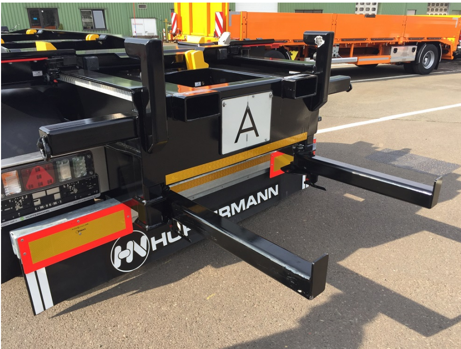
Variante Frontbeladung
