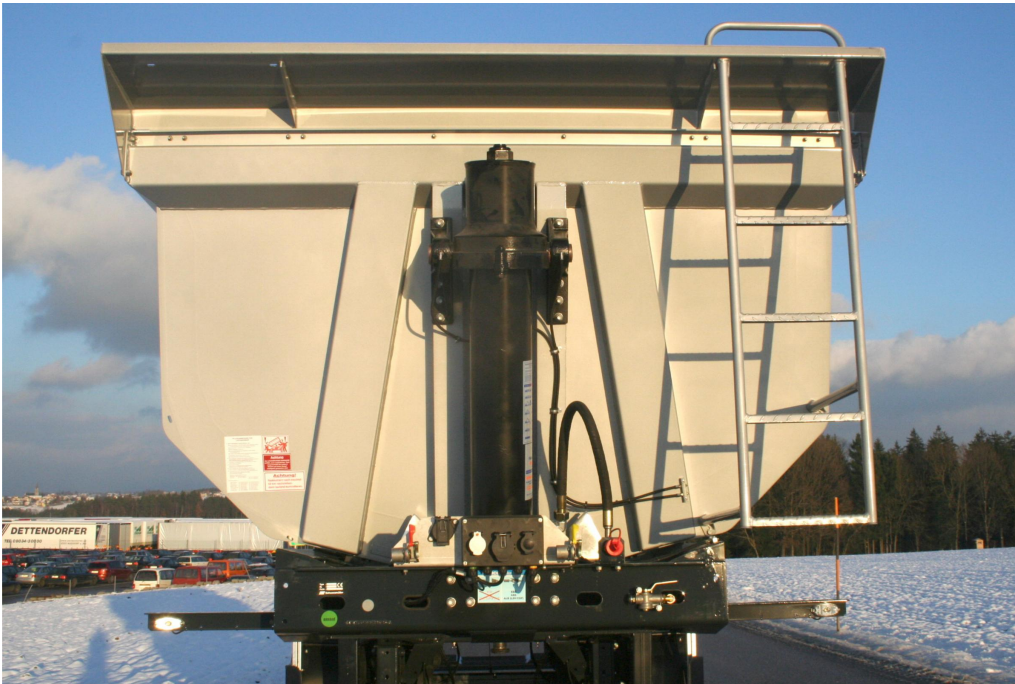
Schräge Vorderwand mit hartverchromtem, qualitativ hochwertigem Frontkippsyliner
