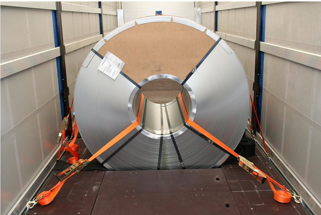
Beladungsbeispiel - Coil-Transport
