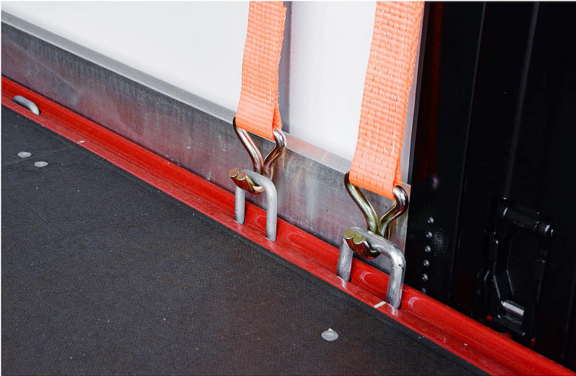
OPTIONAL: Zurrbügel für Coilmulde: Neben den serienmäßigen 2,5 t Zurrbügel gibt es zusätzliche 4 t Zurrbügel für die Coilsicherung.
