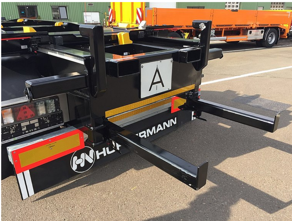
Variante Frontbeladung mit Stapleraufnahme
