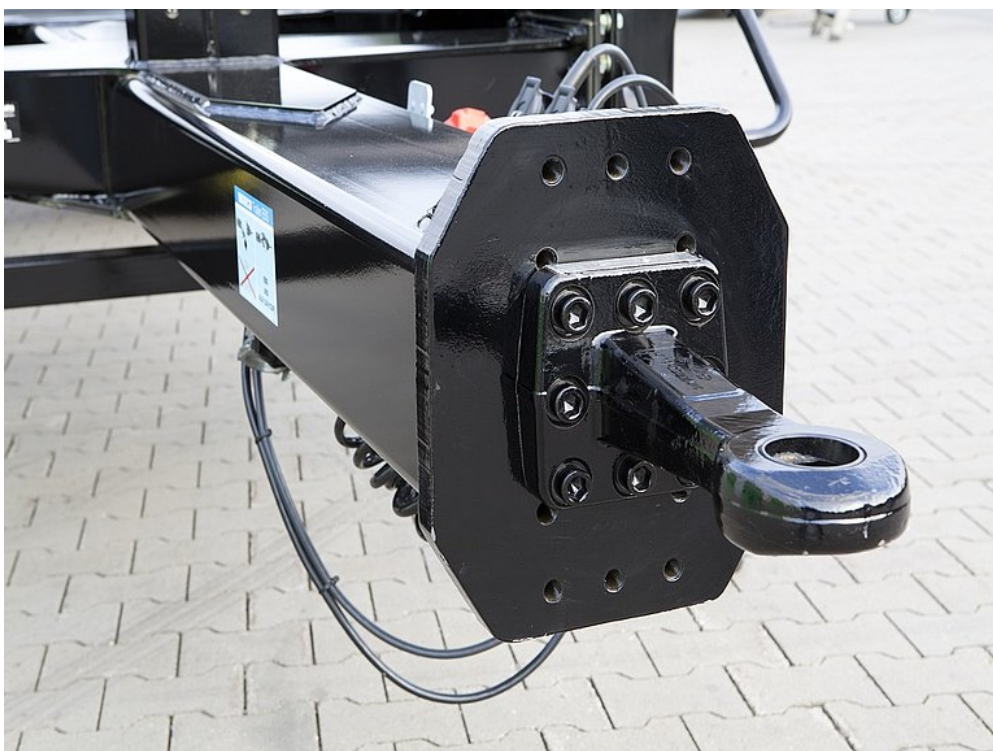
Svařované tažné zařízení s centrální trubicí
