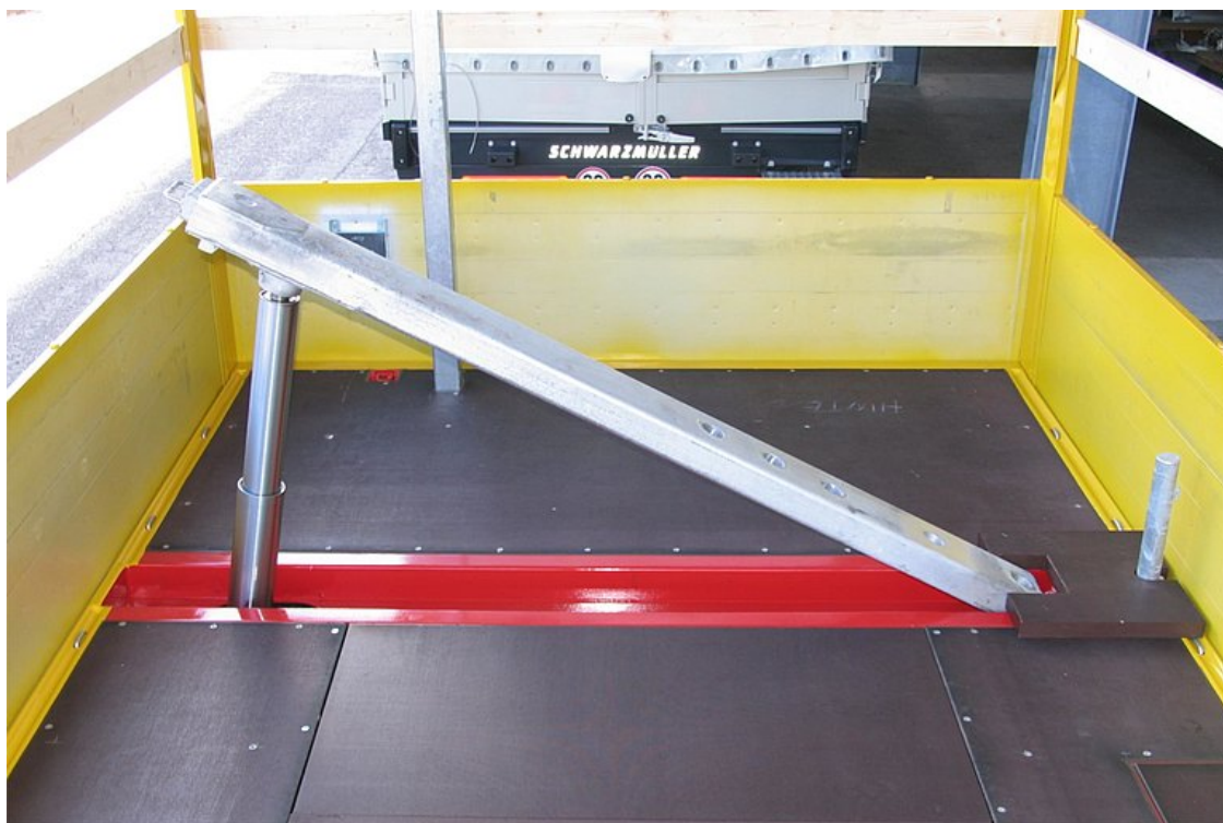
V podlaze jsou zapuštěné profilované opěry, výsuvné prostřednictvím hydraulického čtyřstupňového zdvihacího válce
