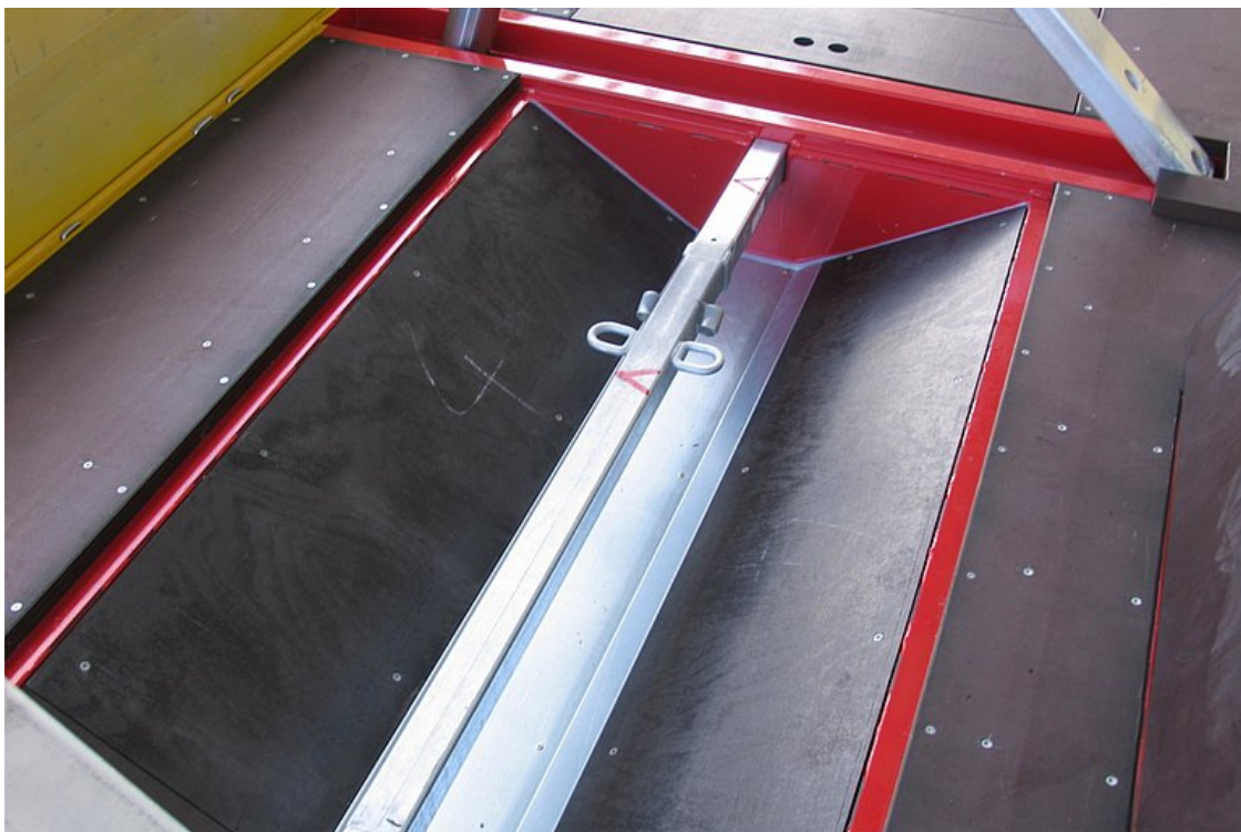
Prohloubené lůžko o užité délce cca 8.000 mm (rozdělené do 3 částí) pro přepravu cívek o průměru 900 mm až max. 2.100 mm
