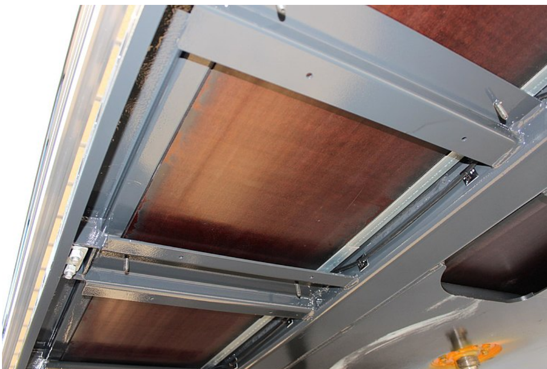
Podlaha z překližky tl. 27 mm, lícující zároveň s vnějším rámem, (zatížení podlahy do 7 t = zatížení na nápravu vysokozdvížného vozíku dle CSC normy)
