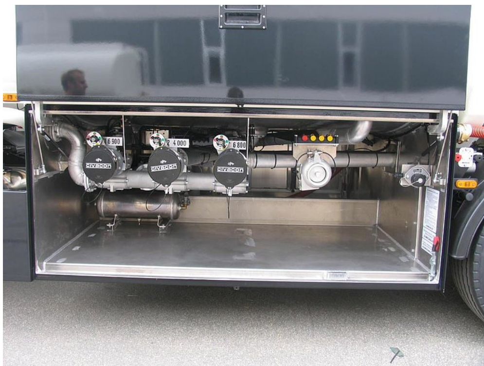
Přístrojová skříň s paralelně otevíraným víkem a s možností umístění jednoho rezervního kola
